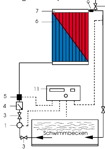
Verrohrungsschema über eigene Pumpe
