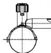
PE 100 RC Anbohrschelle mit Schraubkappe Gasdicht - Unterteil schraubbar SDR 11
