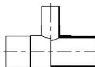
PE 100 RC T-Stück reduziert SDR 11 LANG
