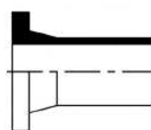
PE 100 RC Vorschweißbund SDR 11 LANG Stumpf + E-Muffenschweißung 26 2 16 8001 ...
