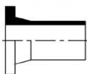
PE 100 RC Vorschweißbund SDR 17 LANG Stumpf + E-Muffenschweißung 26 2 10 8001 ...
