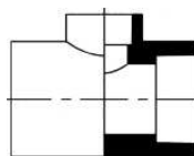
PE 100 T-Stück reduziert SDR 11 MUFFE
