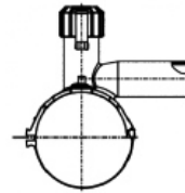
PE 100 RC Anbohrschelle mit Schraubkappe Gasdicht - Unterteil schraubbar
