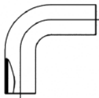
PE 100 RC MULTI-Bogen 90° SDR 17 LANG
