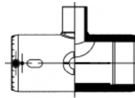
PE 100 RC Heizwendel-T-Stück red. SDR 11
