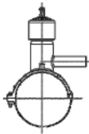
PE 100 RC Druckanbohrventil Messingventil + Schneidschraube
