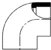
PE 100 RC Winkel 90° SDR 11 MUFFE
