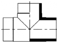
PE 100 RC T-Stück 90° SDR 17 KURZ Schweißstutzen
