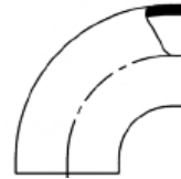
PE 100 RC Bogen 90° SDR 11 KURZ Schweißstutzen
