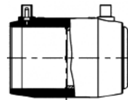
PE 100 RC Heizwendel-Kappe SDR 11
